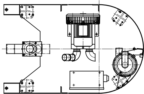
Cross section B-B B-B 断面
